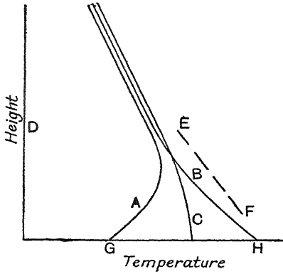
चित्र ४९ (a) — स्थल पर खुले दिन में स्थायित्व में दैनिक परिवर्तन
